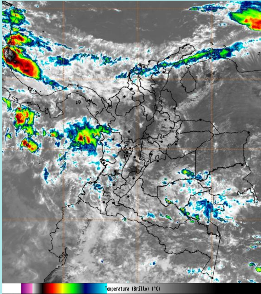
Imagen GOES 19 East Canal Infrarrojo, 14 de septiembre de 2026 - Hora 12:00 HLC. Fuente: https://bart.ideam.gov.co GOES 19
