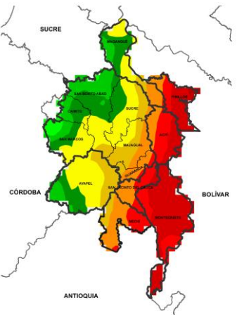
ACUMULADO DEL 16 AL 17 DE AGOSTO
