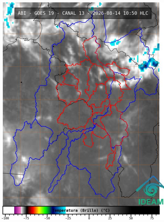
Imagen de satélite IR 10:50 HLC Fuente: IDEAM
