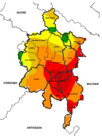
ACUMULADO DEL 17 AL 18 DE AGOSTO
