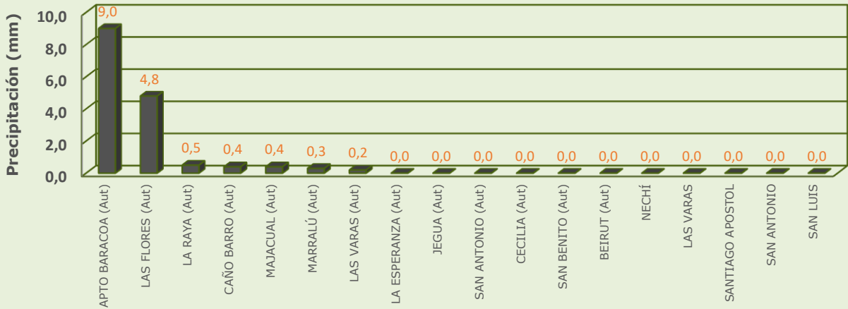
Lluvia registrada el 13 agosto de 2026
