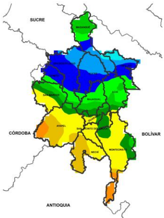
CUMULADO DEL 14 AL 15 DE AGOSTO
