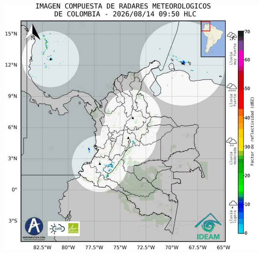
Imagen de radar Barrancabermeja 09:50 HLC Fuente: IDEAM
