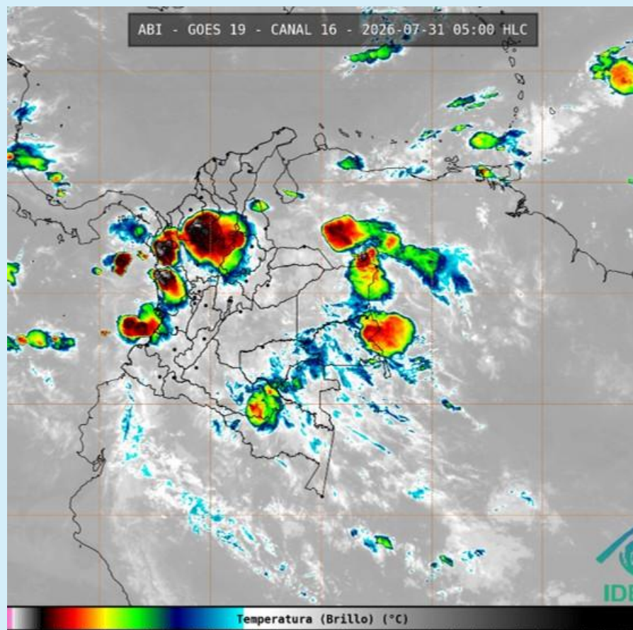
Canal Infrarrojo 30 de julio de 2026 – Hora 05:00 HLC Fuente: GOES 19
