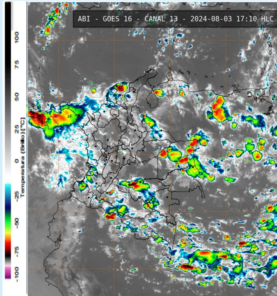
Imagen GOES 16 (East) Canal Infrarrojo | Fuente: GOES-IDEAM 3 de agosto de 2024 - Hora 17:10 HLC
