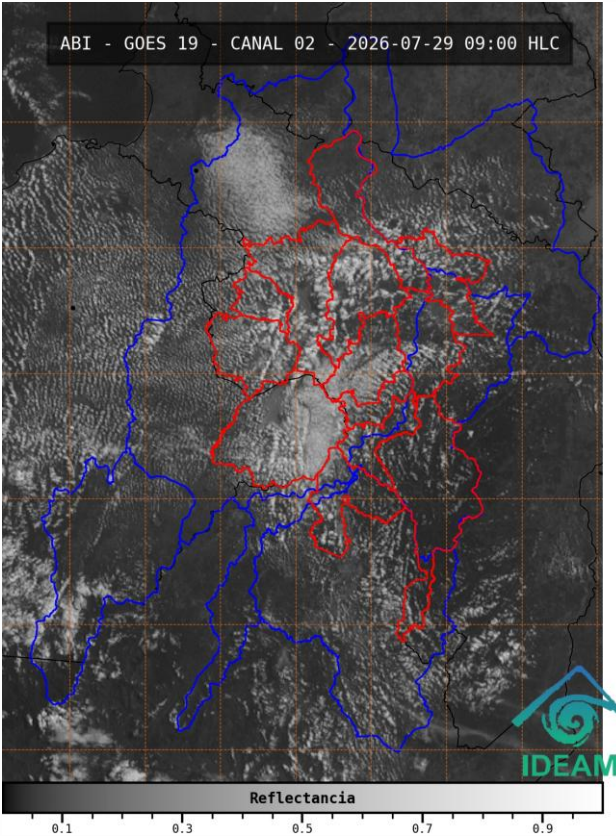
Imagen de satélite VISIBLE 09:00 HLC Fuente: IDEAM
