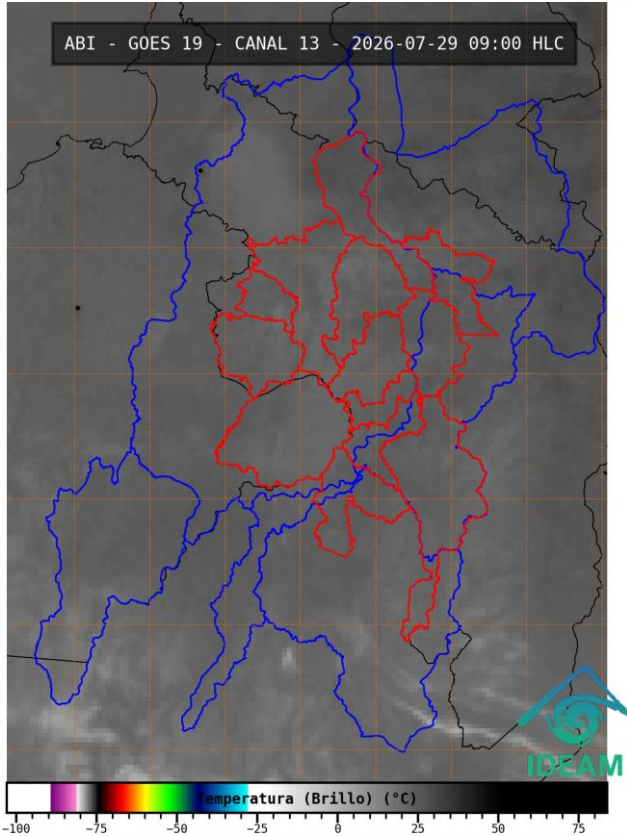
Imagen de satélite IR 09:00 HLC Fuente: IDEAM
