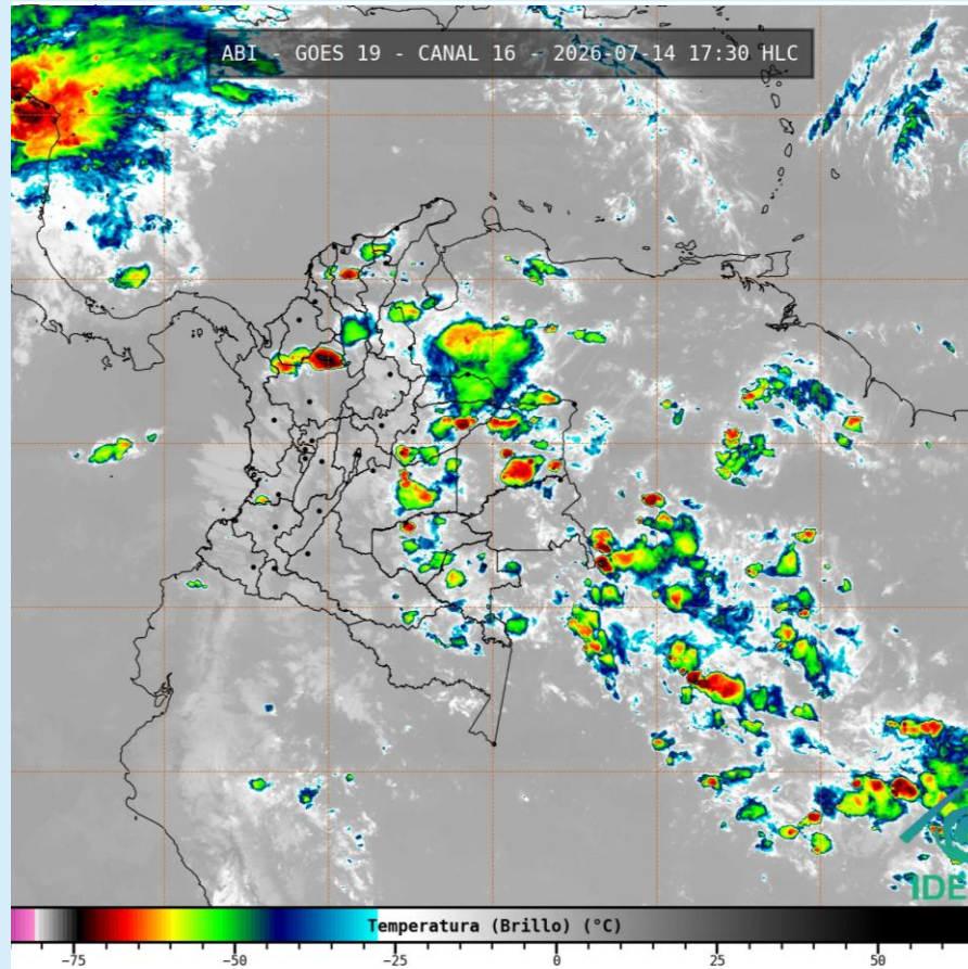
Imagen GOES 19 (East) Canal Infrarrojo 14 de julio de 2026 – Hora 17:40 HLC Fuente: RAMMB CIRA- NOAA
