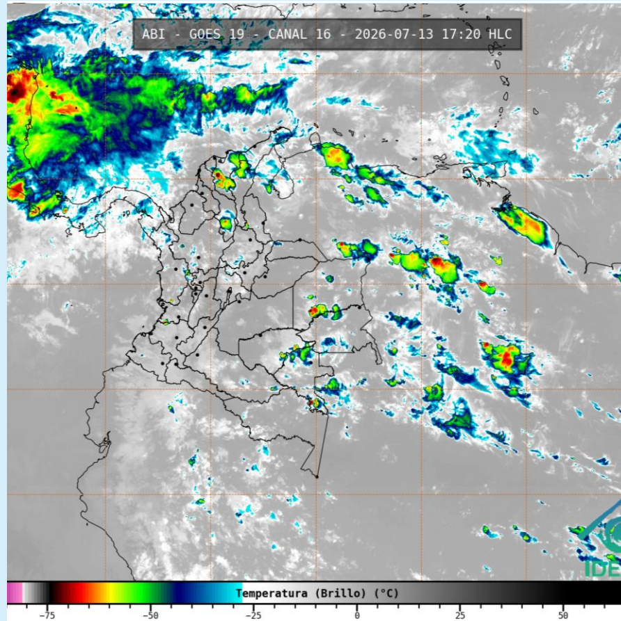
Imagen GOES 19 (East) Canal Infrarrojo 13 de julio de 2026 – Hora 17:20 HLC Fuente: RAMMB CIRA- NOAA
