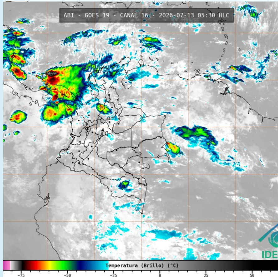
Imagen GOES 19 (East) Canal Infrarrojo 13 de julio de 2026 – Hora 05:30 HLC Fuente: RAMMB CIRA- NOAA
