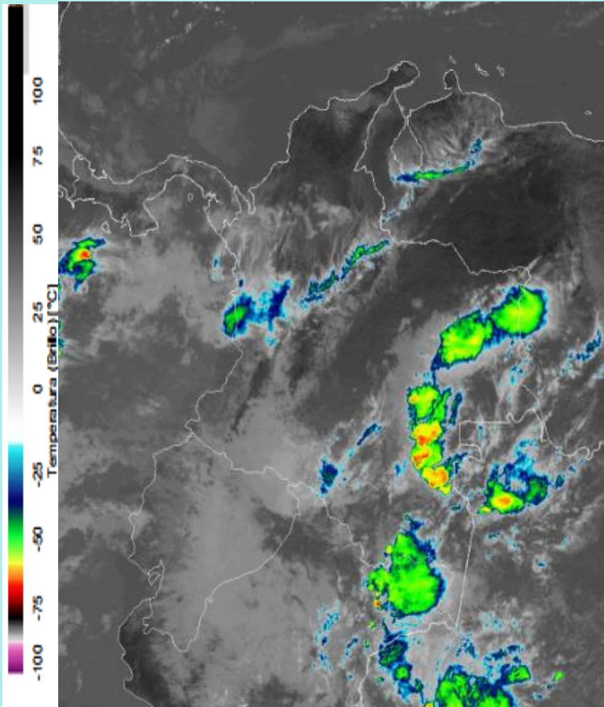
Imagen GOES East Canal Infrarrojo, 15 de marzo de 2024 - Hora 11:20 HLC. Fuente: GOES 16
