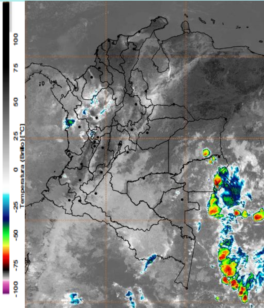
Imagen GOES East Canal Infrarrojo, 13 de marzo de 2024 - Hora 11:30 HLC. Fuente: GOES 16
