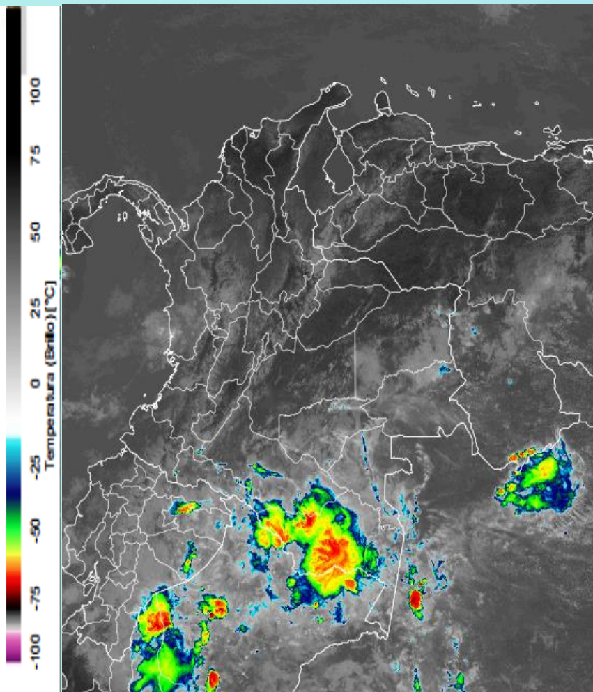
Imagen GOES East Canal Infrarrojo, 6 de marzo de 2024 - Hora 12:00 HLC. Fuente: GOES 16
