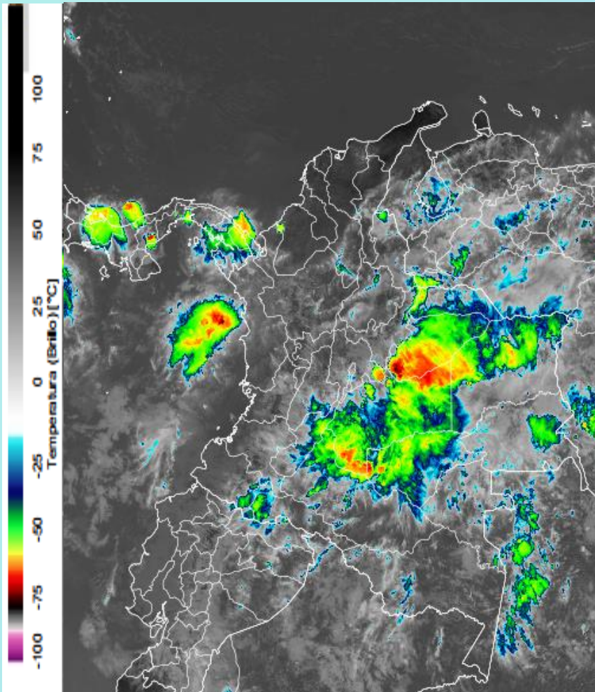
Imagen GOES East Canal Infrarrojo, 18 de mayo de 2024 - Hora 11:40 HLC. Fuente: GOES 16
