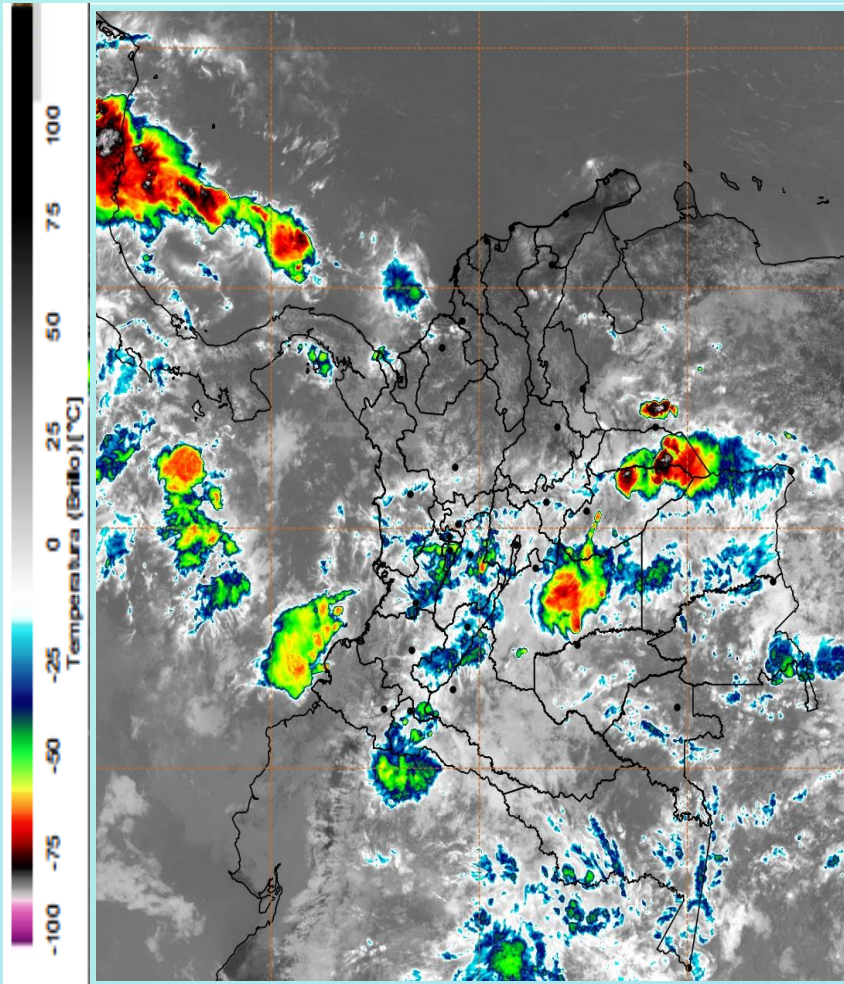
Imagen GOES East Canal Infrarrojo, 16 de mayo de 2024 - Hora 13:40 HLC. Fuente: GOES 16
