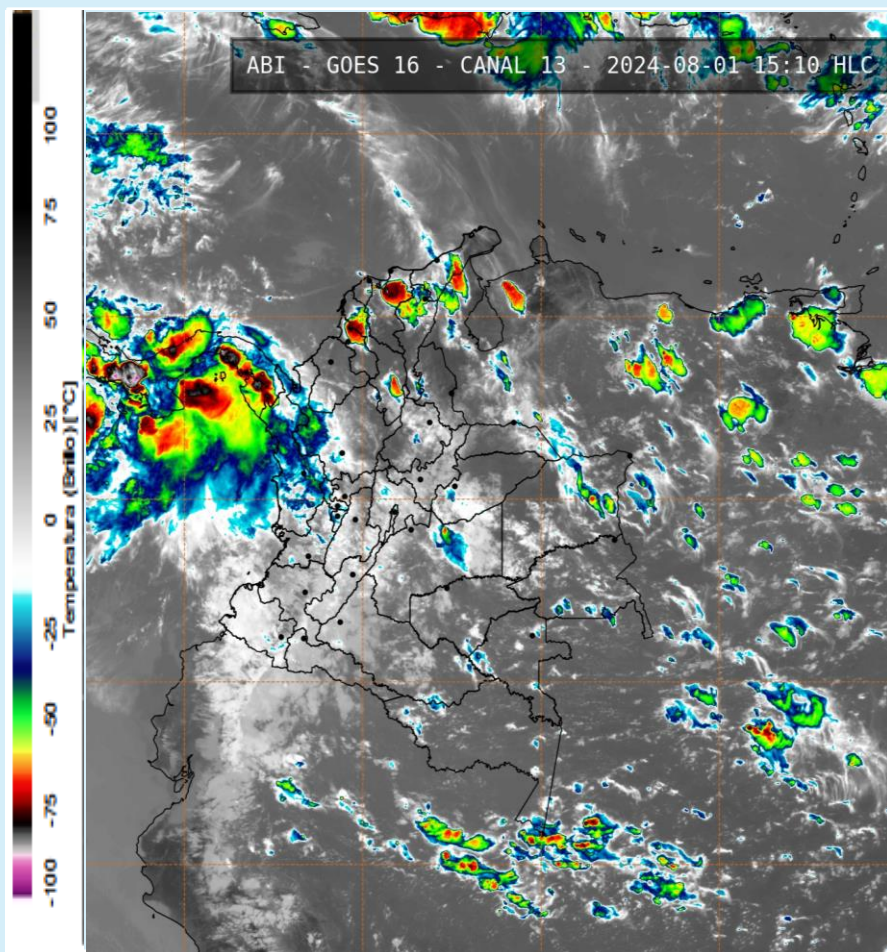
Imagen GOES 16 (East) Canal Infrarrojo | Fuente: GOES-IDEAM 1 de agosto de 2024 - Hora 15:10 HLC
