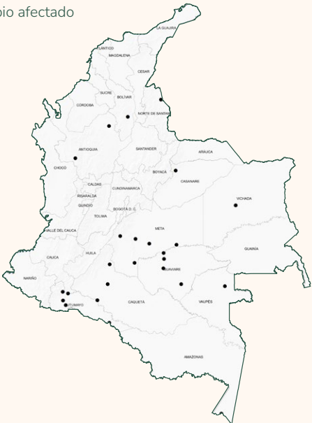
Distribución de municipios con mayor cantidad de Detecciones Tempranas de Deforestación (DTD), cuarto trimestre de 2025
