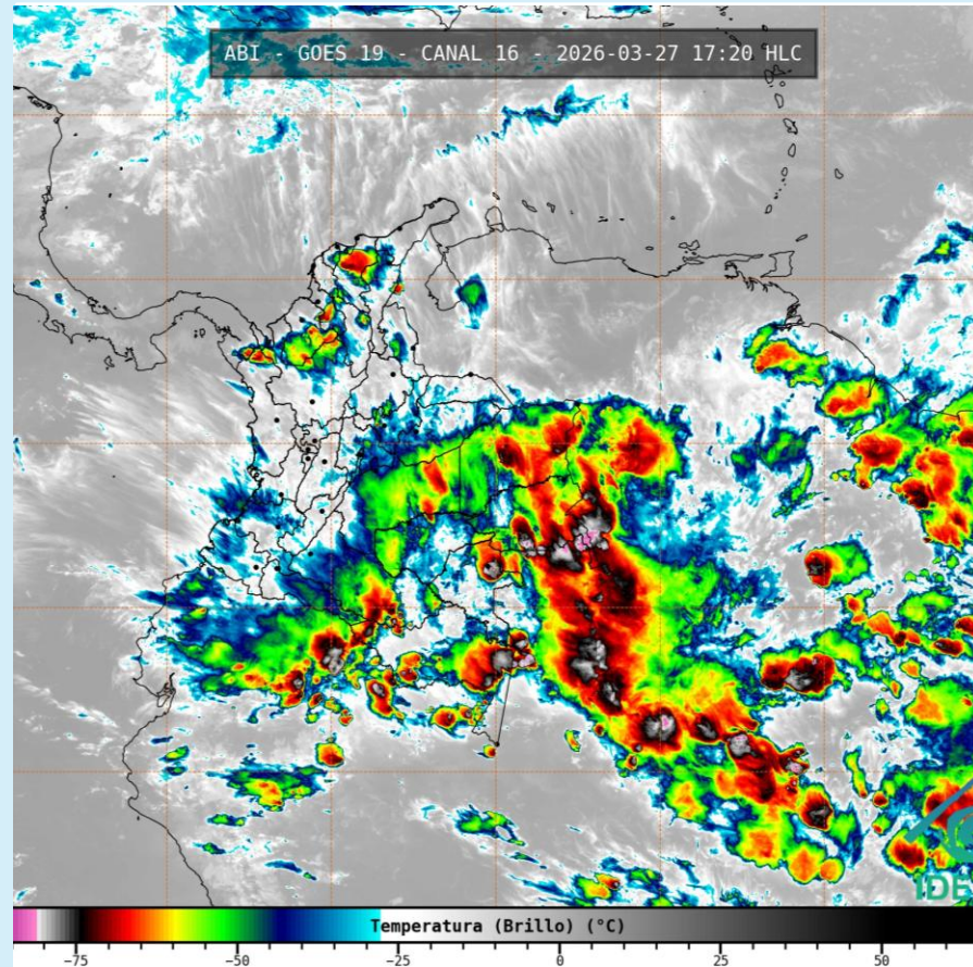
Imagen GOES 19 (East) Canal Infrarrojo 27 de marzo de 2026 – Hora 17:20 HLC Fuente: IDEAM - GOES 19
