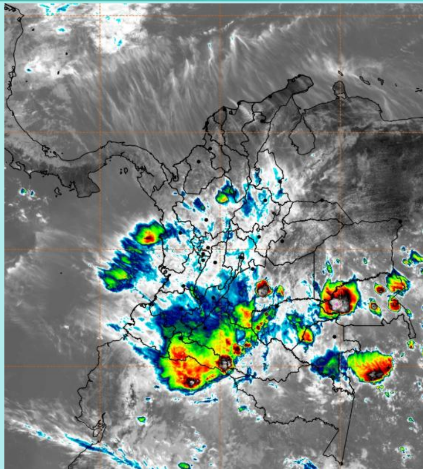
Imagen GOES 19 East Canal Infrarrojo, 27 de marzo de 2026 - Hora 12:00 HLC. Fuente: https://bart.ideam.gov.co GOES 19
