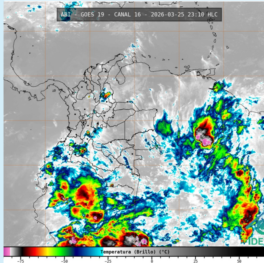
Imagen GOES 19 (East) Canal Infrarrojo 25 de marzo de 2026 – Hora 23:10 HLC Fuente: IDEAM - GOES 19
