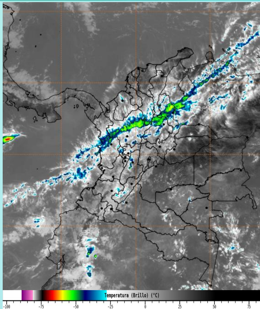
Imagen GOES 19 East Canal Infrarrojo, 24 de marzo de 2026 - Hora 12:00 HLC. Fuente: https://bart.ideam.gov.co GOES 19
