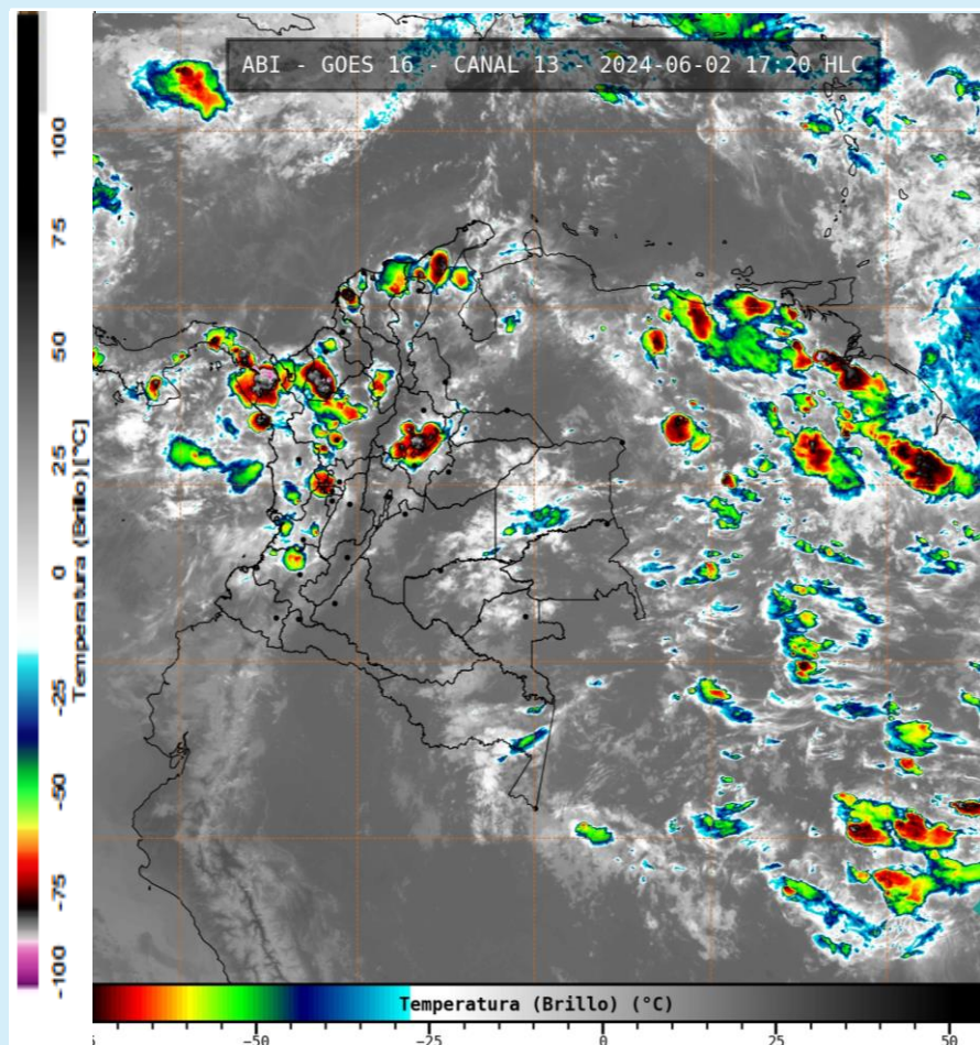
Imagen GOES 16 (East) Canal Infrarrojo | Fuente: GOES-IDEAM 2 de junio de 2024 - Hora 17:20 HLC
