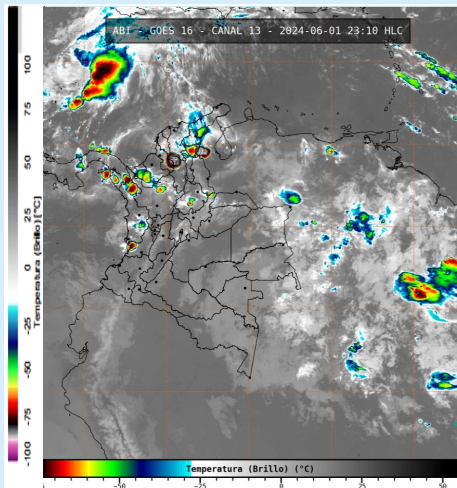
Imagen GOES 16 (East) Canal Infrarrojo | Fuente: GOES-IDEAM 1 de junio de 2024 - Hora 23:10 HLC
