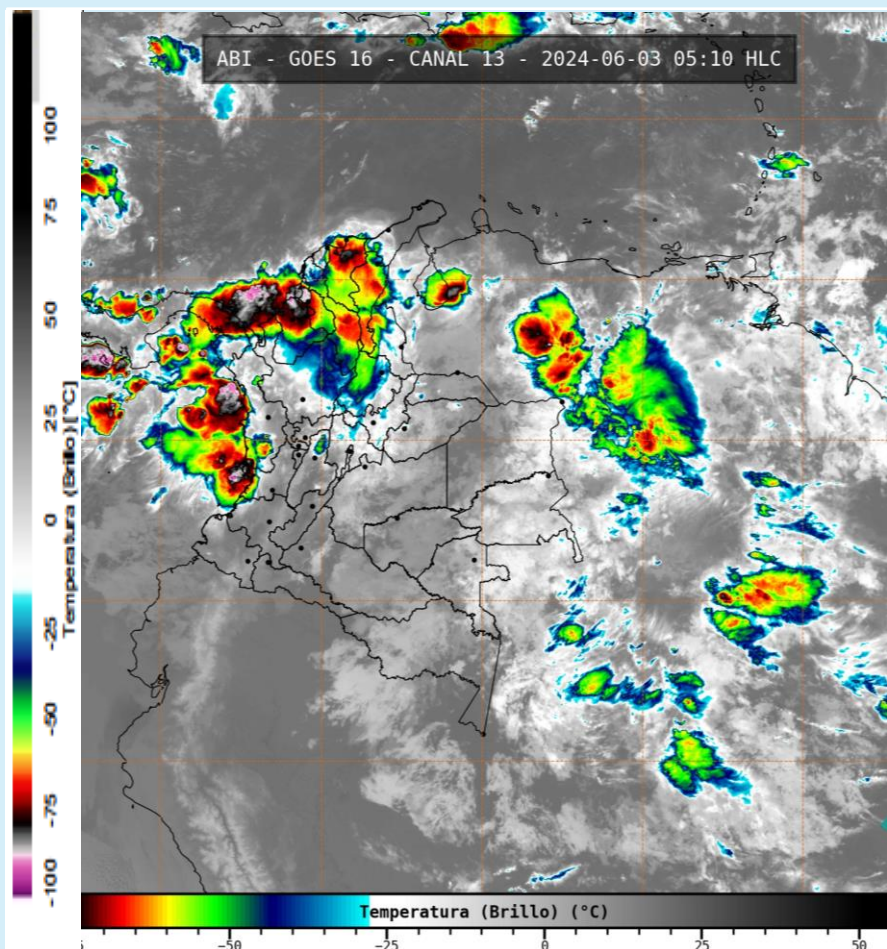
Imagen GOES 16 (East) Canal Infrarrojo | Fuente: GOES-IDEAM 3 de junio de 2024 - Hora 05:10 HLC
