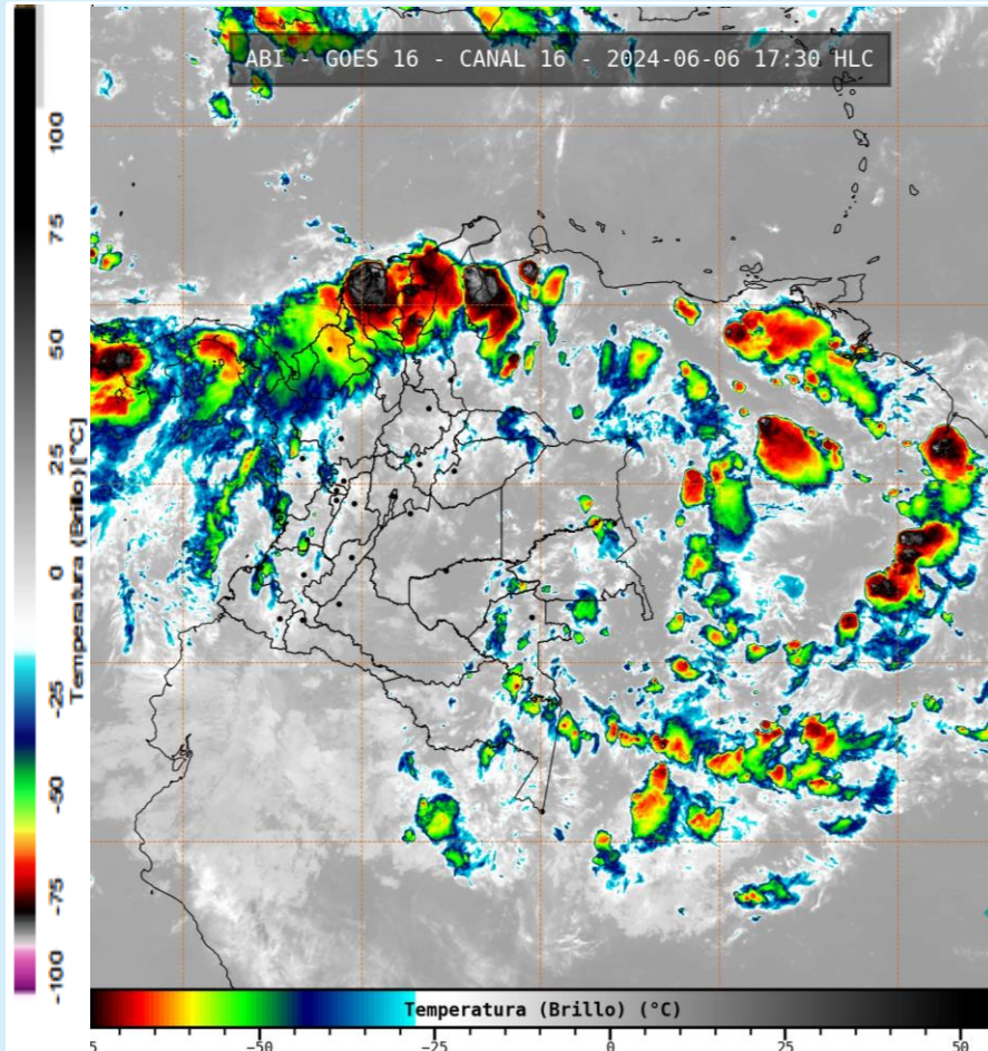
Imagen GOES 16 (East) Canal Infrarrojo | Fuente: GOES-IDEAM 6 de junio de 2024 - Hora 17:30 HLC
