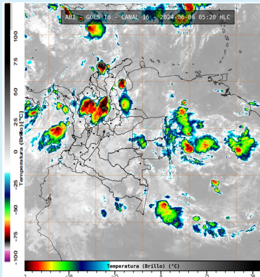
Imagen GOES 16 (East) Canal Infrarrojo | Fuente: GOES-IDEAM 6 de junio de 2024 - Hora 05:20 HLC
