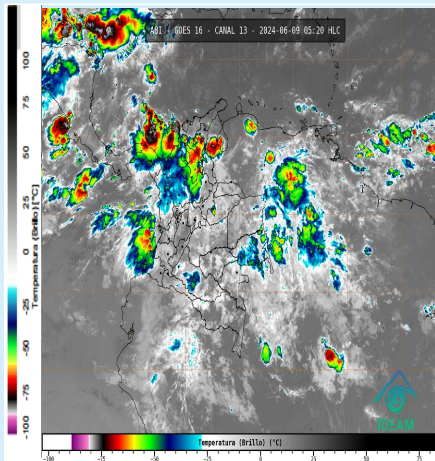
Imagen GOES 16 (East) Canal Infrarrojo | Fuente: GOES-IDEAM 9 de junio de 2024 - Hora 05:20 HLC
