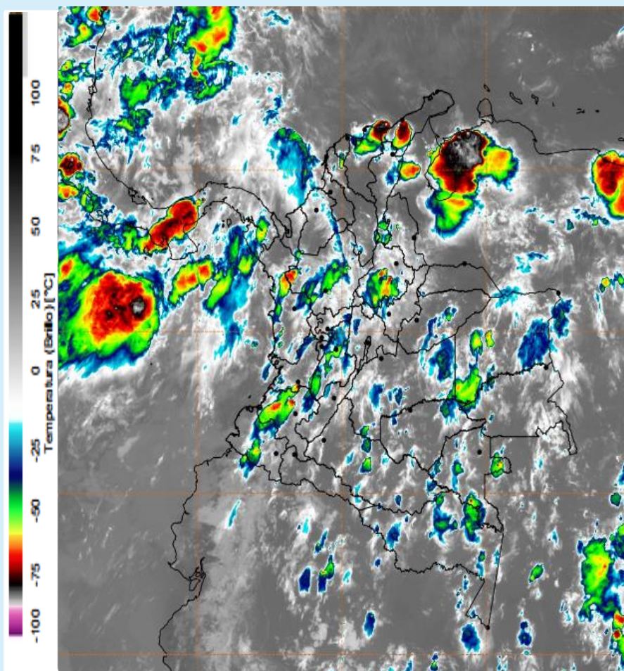
Imagen GOES 16 (East) Canal Infrarrojo | Fuente: GOES-IDEAM 10 de junio de 2024 - Hora 23:20 HLC
