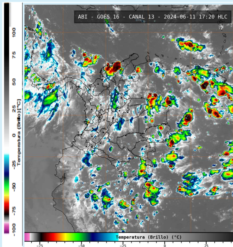
Imagen GOES 16 (East) Canal Infrarrojo | Fuente: GOES-IDEAM 11 de junio de 2024 - Hora 17:20 HLC
