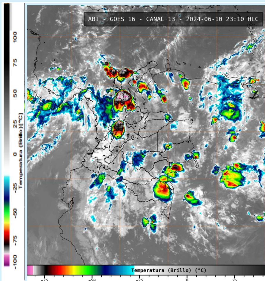
Imagen GOES 16 (East) Canal Infrarrojo | Fuente: GOES-IDEAM 10 de junio de 2024 - Hora 23:10 HLC
