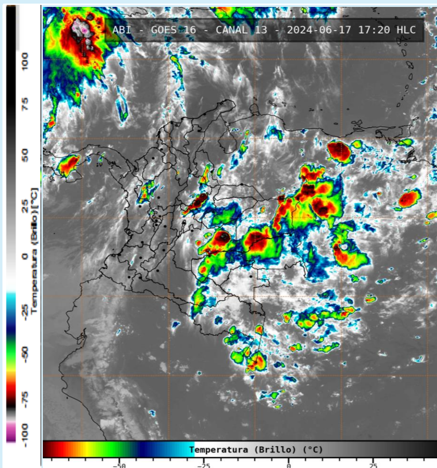
Imagen GOES 16 (East) Canal Infrarrojo | Fuente: GOES-IDEAM 17 de junio de 2024 - Hora 17:20 HLC
