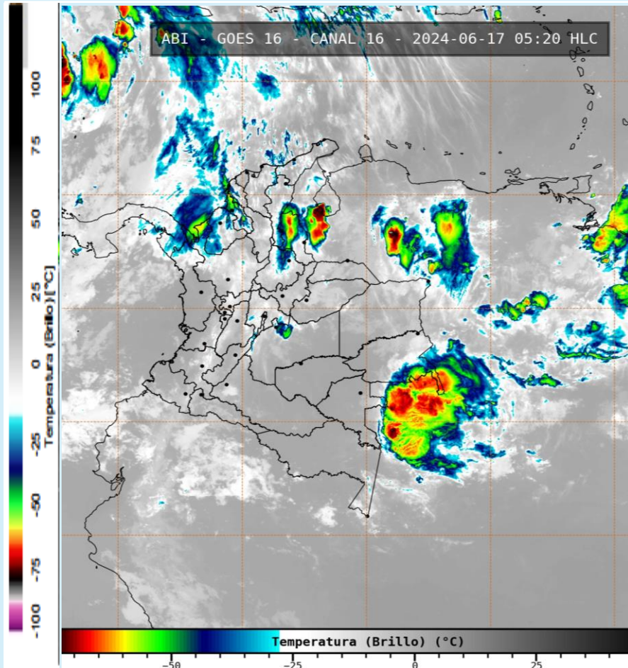
Imagen GOES 16 (East) Canal Infrarrojo | Fuente: GOES-IDEAM 17 de junio de 2024 - Hora 05:20 HLC
