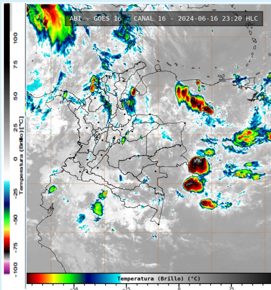
Imagen GOES 16 (East) Canal Infrarrojo | Fuente: GOES-IDEAM 16 de junio de 2024 - Hora 23:20 HLC
