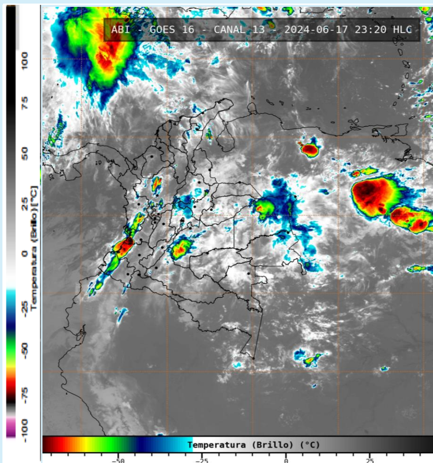
Imagen GOES 16 (East) Canal Infrarrojo | Fuente: GOES-IDEAM 17 de junio de 2024 - Hora 23:20 HLC
