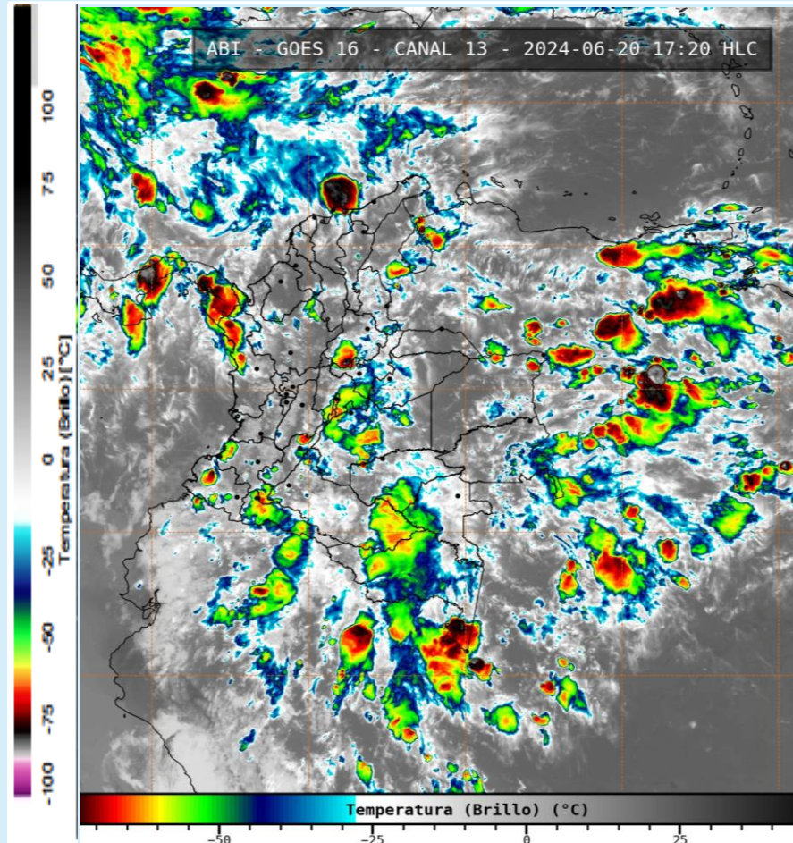
Imagen GOES 16 (East) Canal Infrarrojo | Fuente: GOES-IDEAM 20 de junio de 2024 - Hora 17:20 HLC
