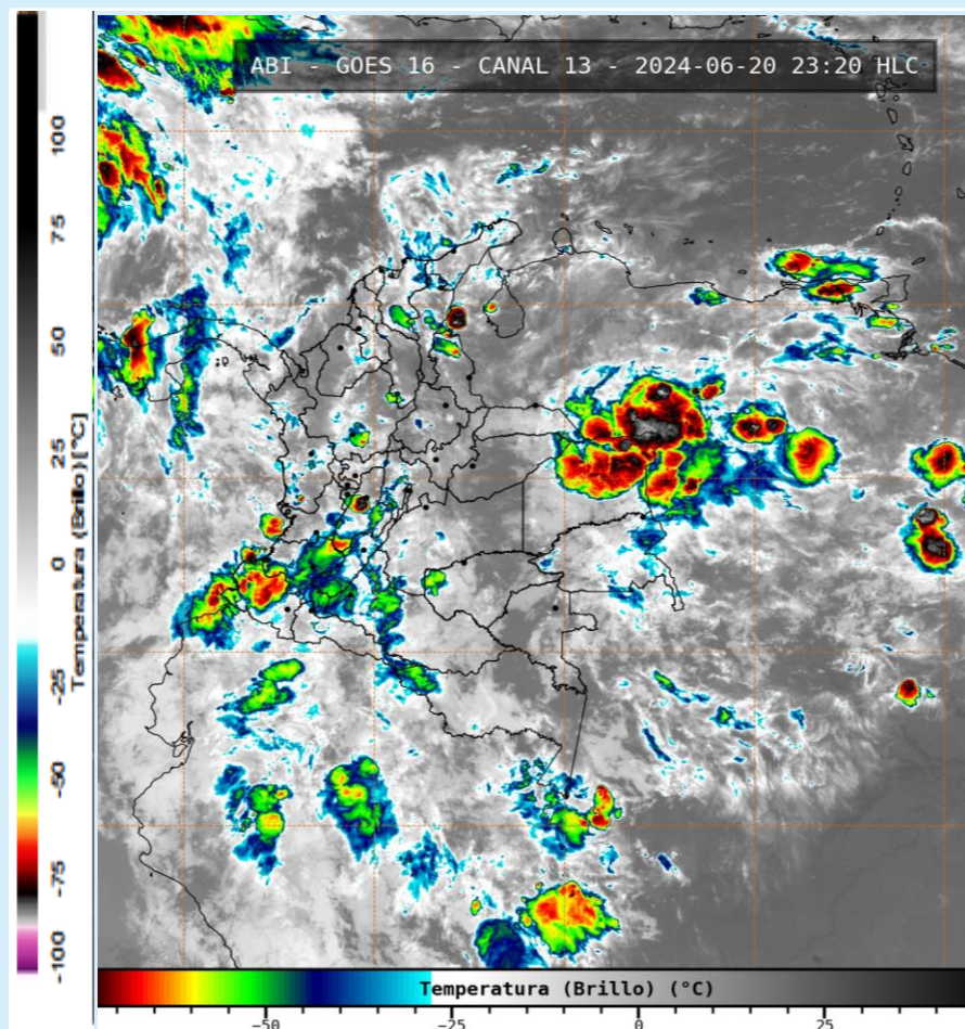
Imagen GOES 16 (East) Canal Infrarrojo | Fuente: GOES-IDEAM 20 de junio de 2024 - Hora 23:20 HLC
