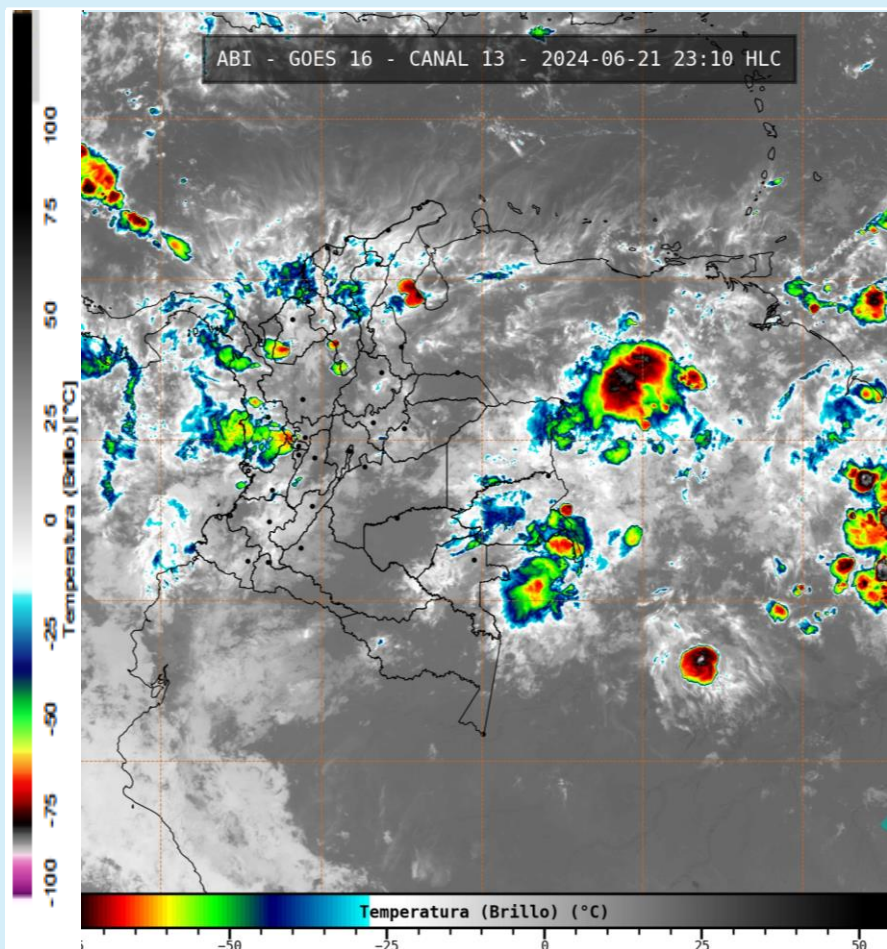
Imagen GOES 16 (East) Canal Infrarrojo | Fuente: GOES-IDEAM 21 de junio de 2024 - Hora 23:10 HLC
