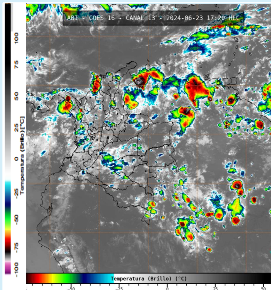
Imagen GOES 16 (East) Canal Infrarrojo | Fuente: GOES-IDEAM 23 de junio de 2024 - Hora 17:20 HLC
