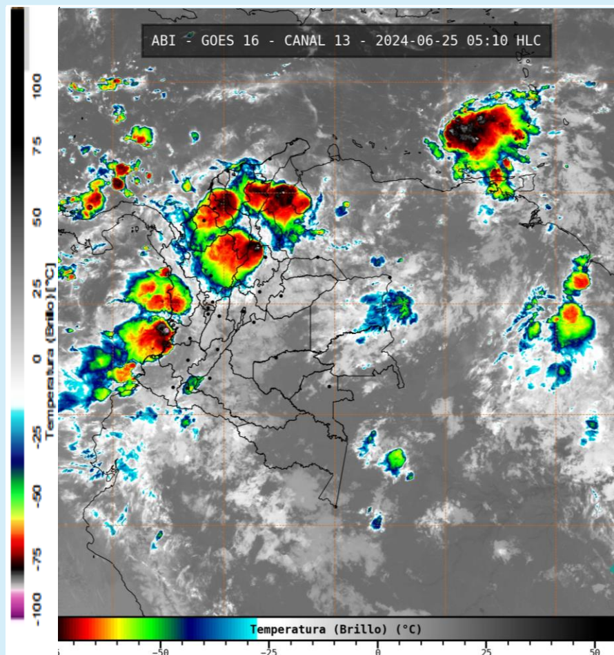
Imagen GOES 16 (East) Canal Infrarrojo | Fuente: GOES-IDEAM 25 de junio de 2024 - Hora 05:10 HLC
