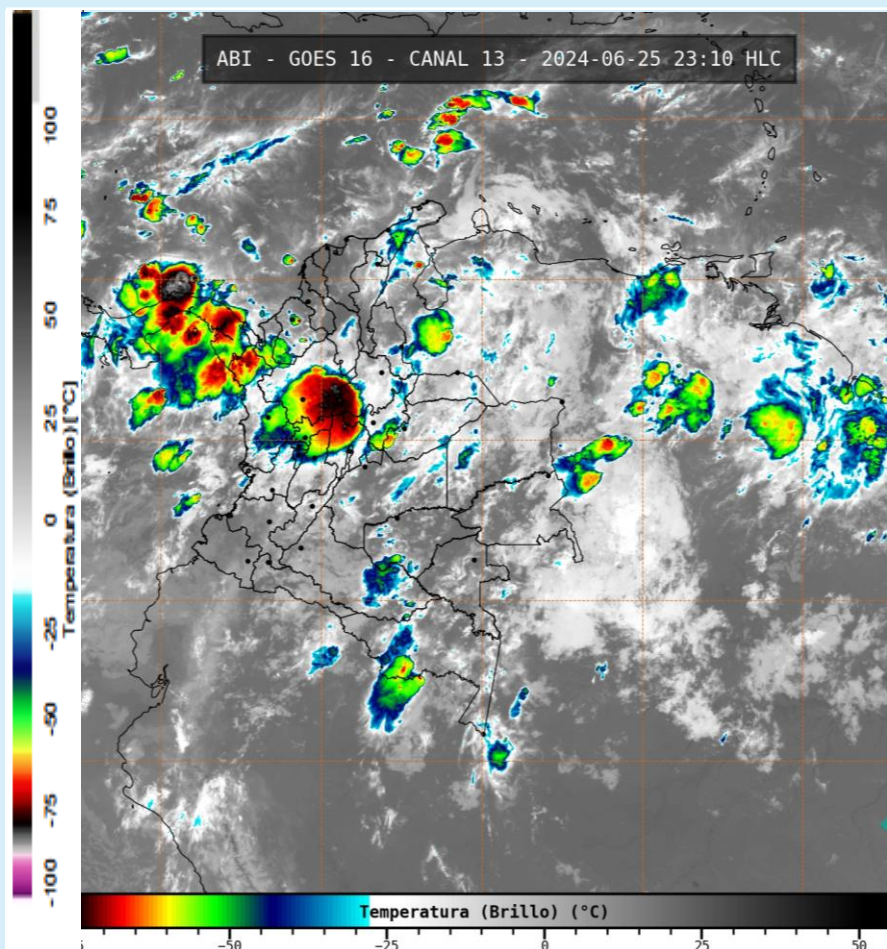
Imagen GOES 16 (East) Canal Infrarrojo | Fuente: GOES-IDEAM 25 de junio de 2024 - Hora 23:10 HLC
