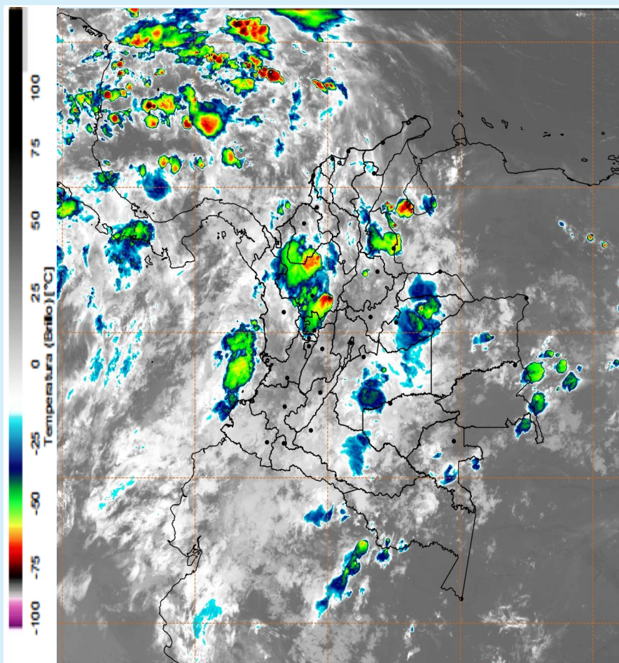
Imagen GOES 16 (East) Canal Infrarrojo | Fuente: GOES-IDEAM 26 de junio de 2024 - Hora 23:20 HLC
