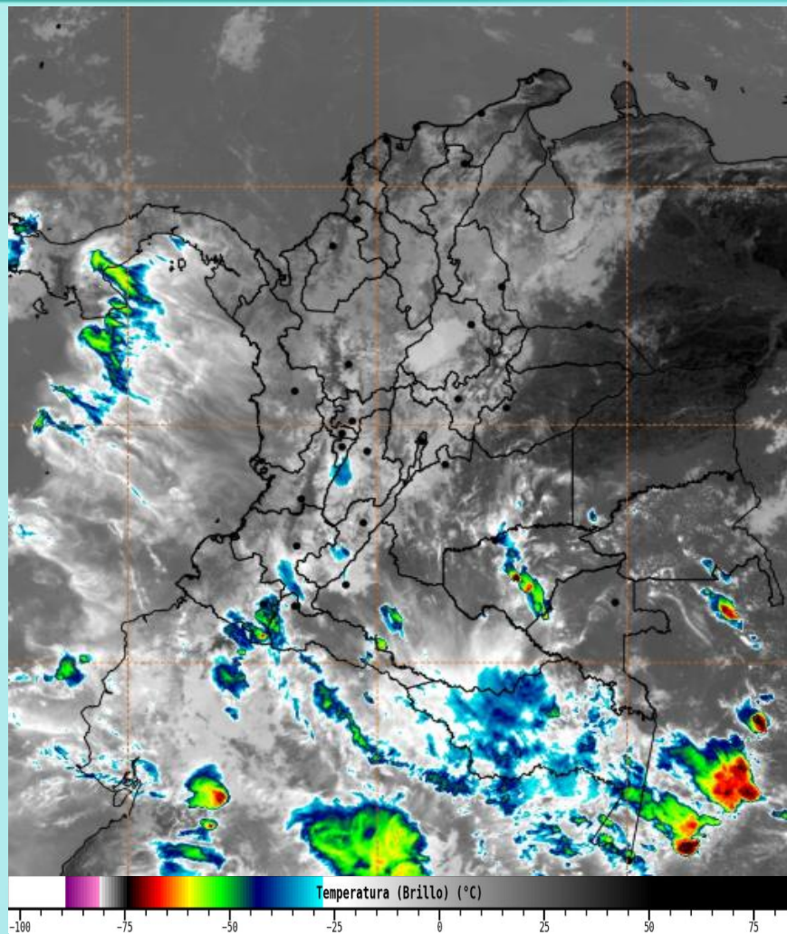
Imagen GOES 19 East Canal Infrarrojo, 23 de marzo de 2026 - Hora 12:10 HLC. Fuente: https://bart.ideam.gov.co GOES 19
