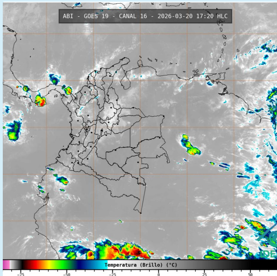
Imagen GOES 19 (East) Canal Infrarrojo 20 de marzo de 2026 – Hora 17:20 HLC Fuente: IDEAM - GOES 19
