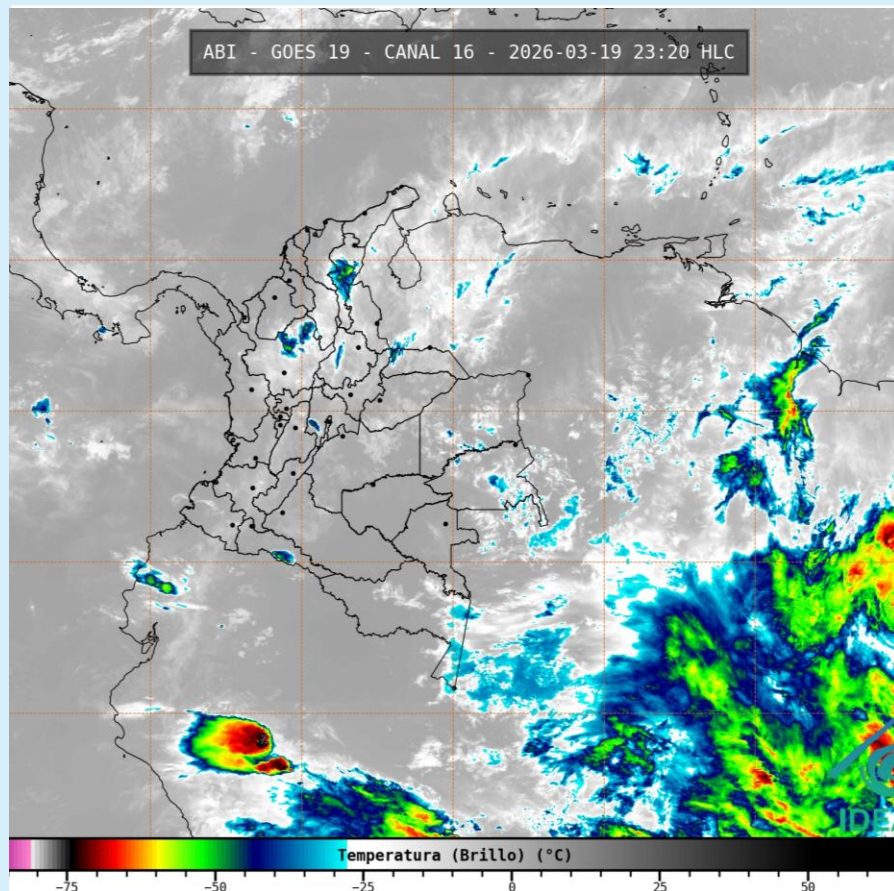
Imagen GOES 19 (East) Canal Infrarrojo 19 de marzo de 2026 – Hora 23:20 HLC Fuente: IDEAM - GOES 19
