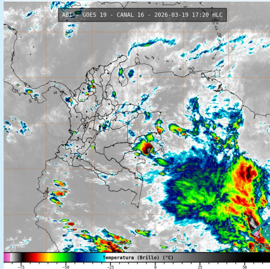
Imagen GOES 19 (East) Canal Infrarrojo 19 de marzo de 2026 – Hora 17:20 HLC Fuente: IDEAM - GOES 19
