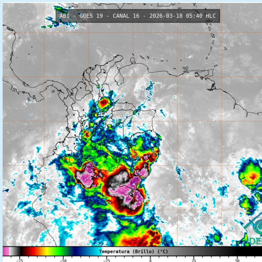
Imagen GOES 19 (East) Canal Infrarrojo 18 de marzo de 2026 – Hora 05:40 HLC Fuente: IDEAM - GOES 19
