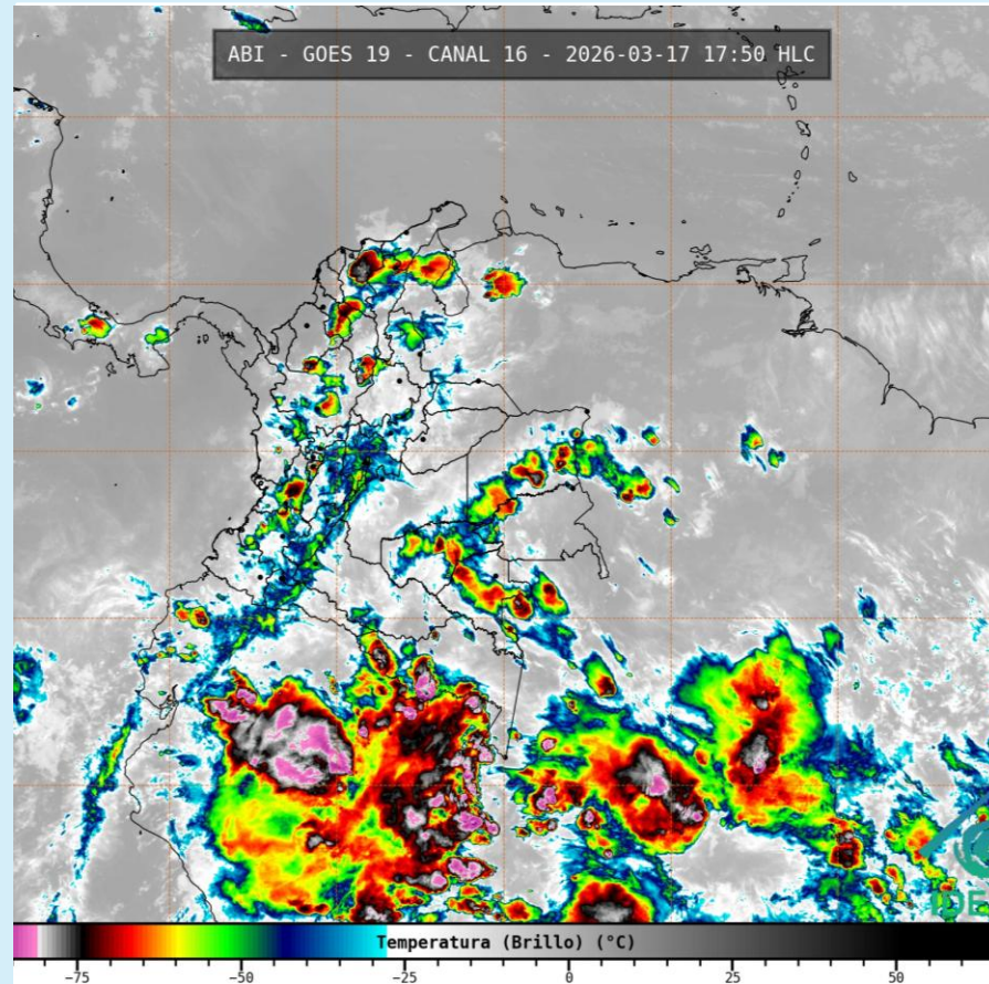
Imagen GOES 19 (East) Canal Infrarrojo 17 de marzo de 2026 – Hora 17:50 HLC Fuente: IDEAM - GOES 19
