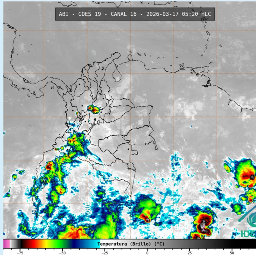
Imagen GOES 19 (East) Canal Infrarrojo 17 de marzo de 2026 – Hora 05:20 HLC Fuente: IDEAM - GOES 19
