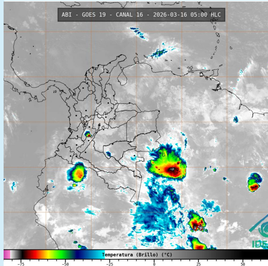
Imagen GOES 19 (East) Canal Infrarrojo 16 de marzo de 2026 – Hora 05:00 HLC Fuente: IDEAM - GOES 19
