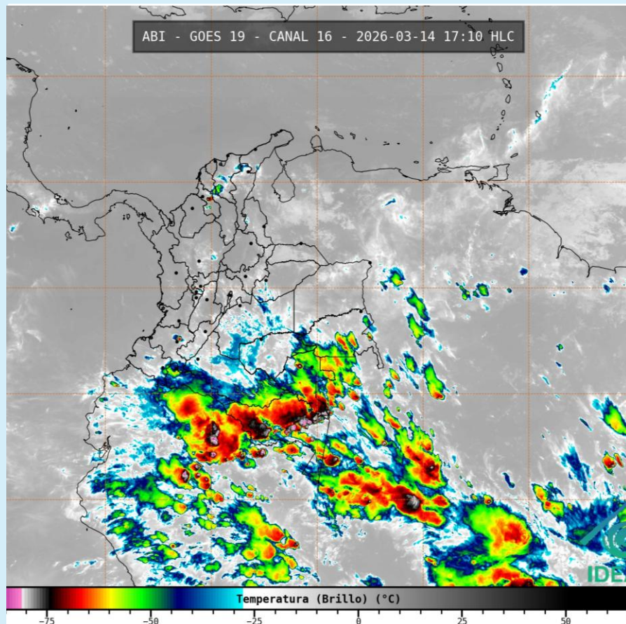
Imagen GOES 19 (East) Canal Infrarrojo 14 de marzo de 2026 – Hora 17:10 HLC Fuente: IDEAM - GOES 19
