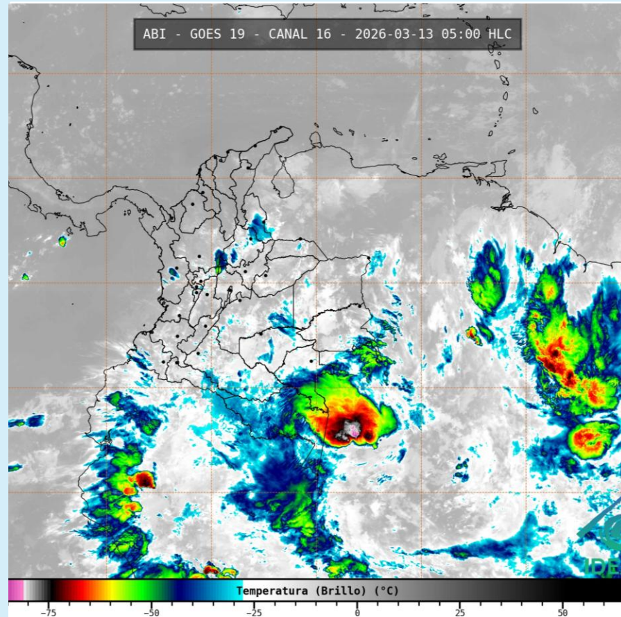
Imagen GOES 19 (East) Canal Infrarrojo 13 de marzo de 2026 – Hora 05:00 HLC Fuente: IDEAM - GOES 19
