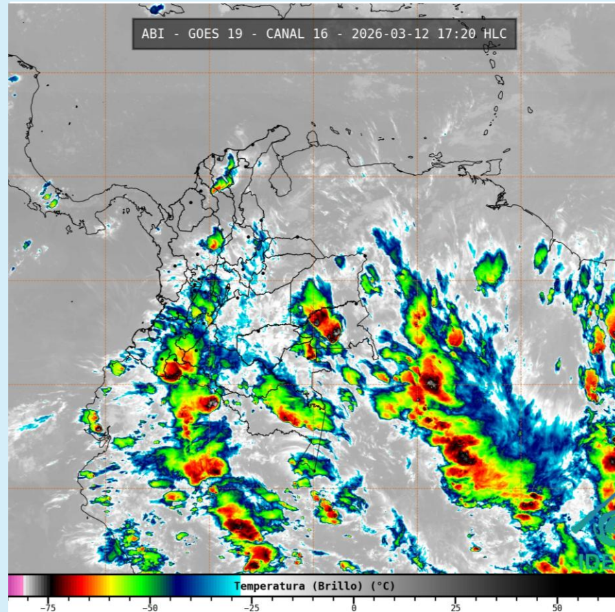
Imagen GOES 19 (East) Canal Infrarrojo 12 de marzo de 2026 – Hora 17:20 HLC Fuente: IDEAM - GOES 19
